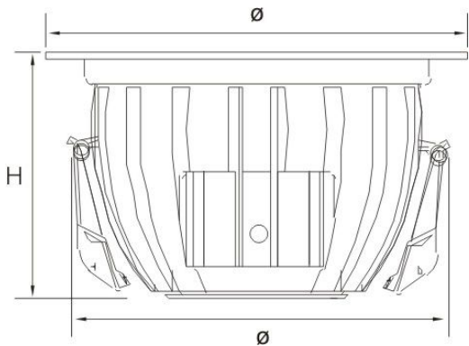
●尺寸图 < mm>
