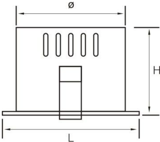
●尺寸图 < mm>
