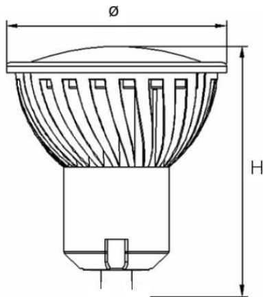
●尺寸图 < mm>
