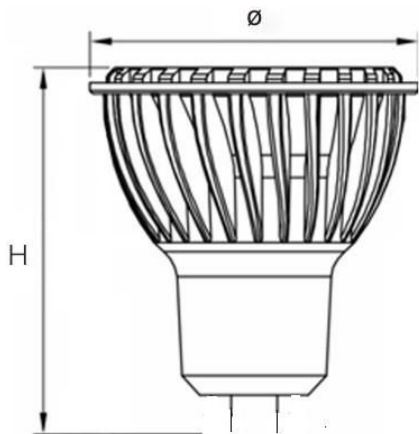
●尺寸图 < mm>
