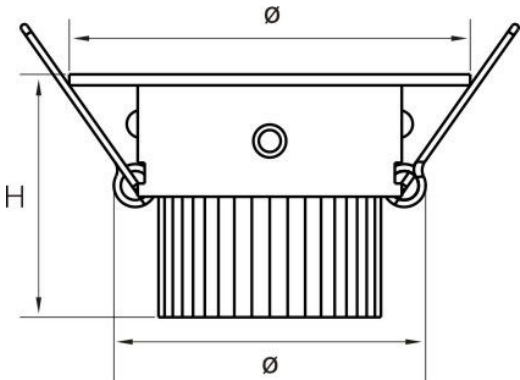
● 尺寸图 < mm >
